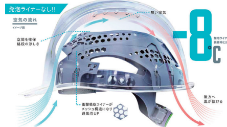
SYA-CV型遮熱エアロメッシュ
